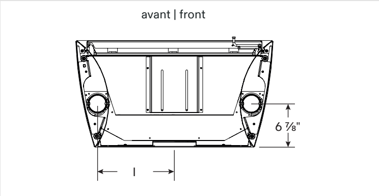
vue de dessous | bottom view
