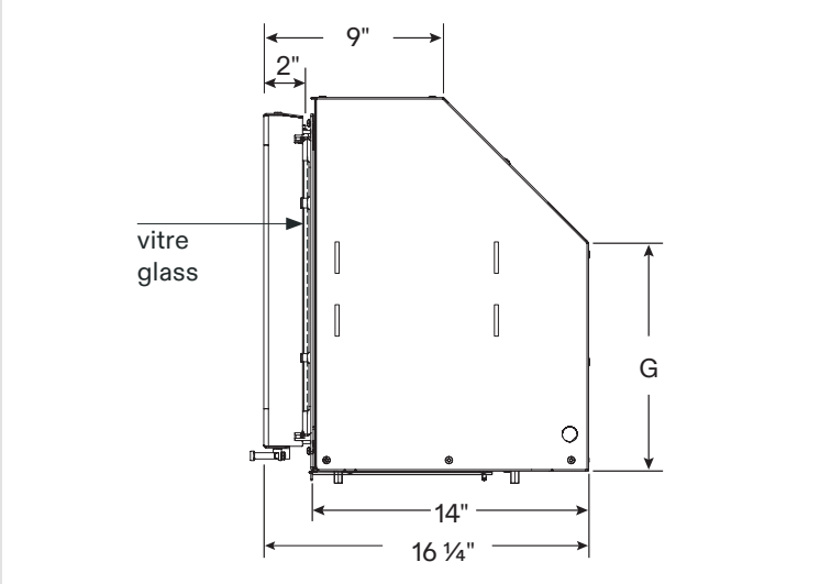
vue de côté | side view
