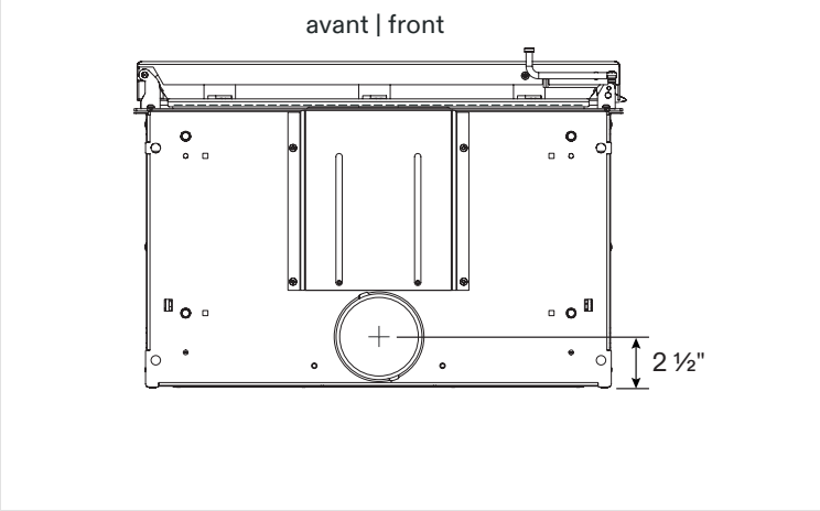
vue de dessous | bottom view
