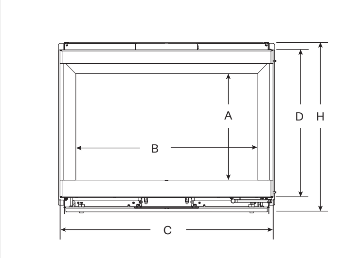
vue de face | front view
